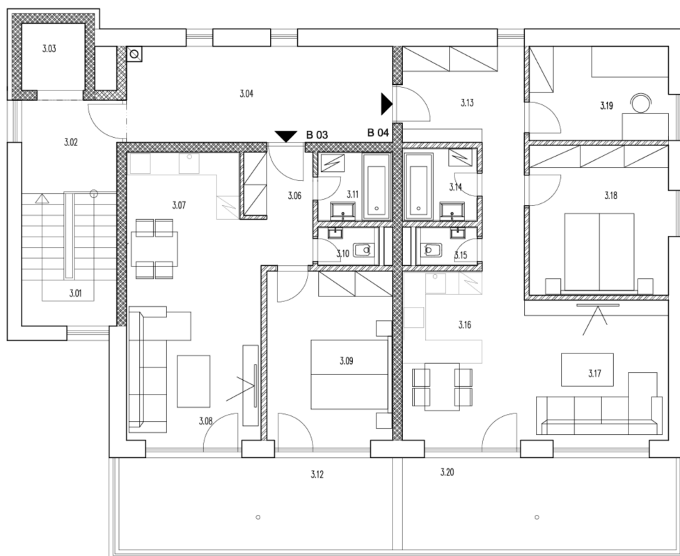
Kanianka - Pánský háj - Byty - Blok 1B - 3.NP
