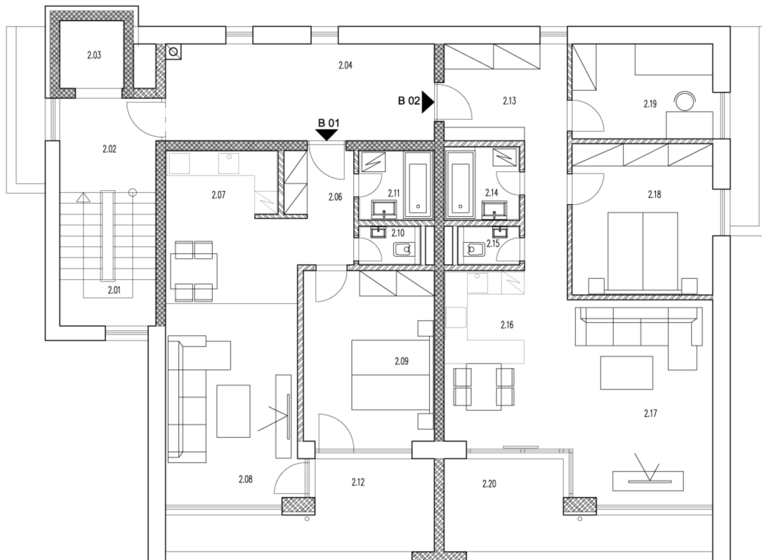
Kanianka - Pánský háj - Byty - Blok 1B - 2.NP
